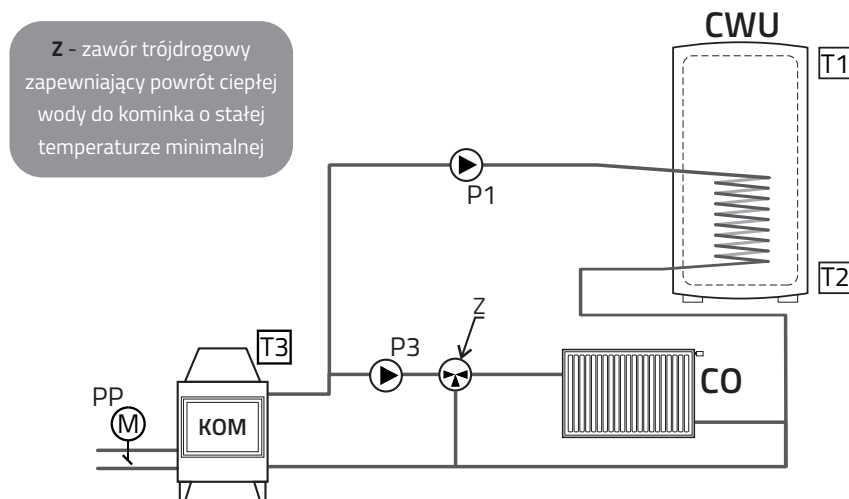
Rys. 1a Podstawowy układ pracy regulatora
