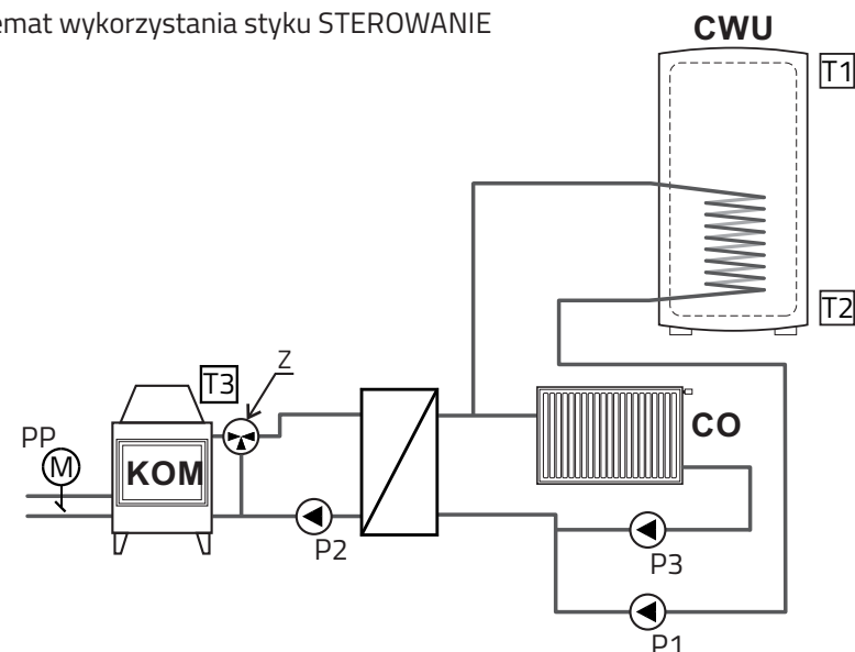
Schemat podłączenia styku STER
