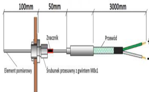
Termopara typu K
